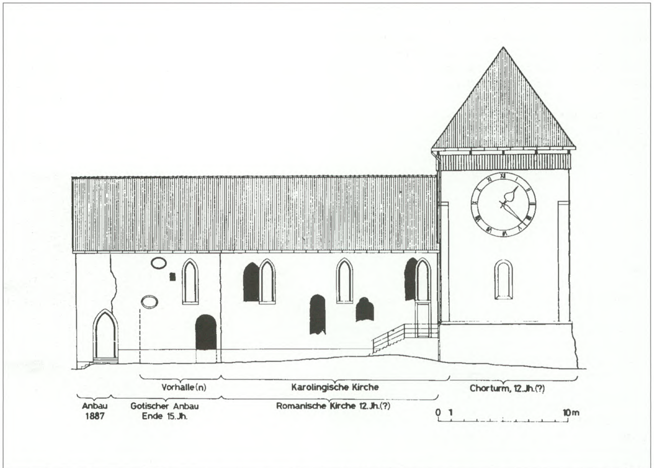
Die Südseite der Kirche Illnau. Dunkel eingezeichnet sind frühere Fensteröffnungen. Der Kernbau ist die wahrscheinlich Mitte des 8. Jahrhunderts entstandene Karolingische Kirche (6. Bericht der Zürcher Denkmalpflege, 1968/69).
