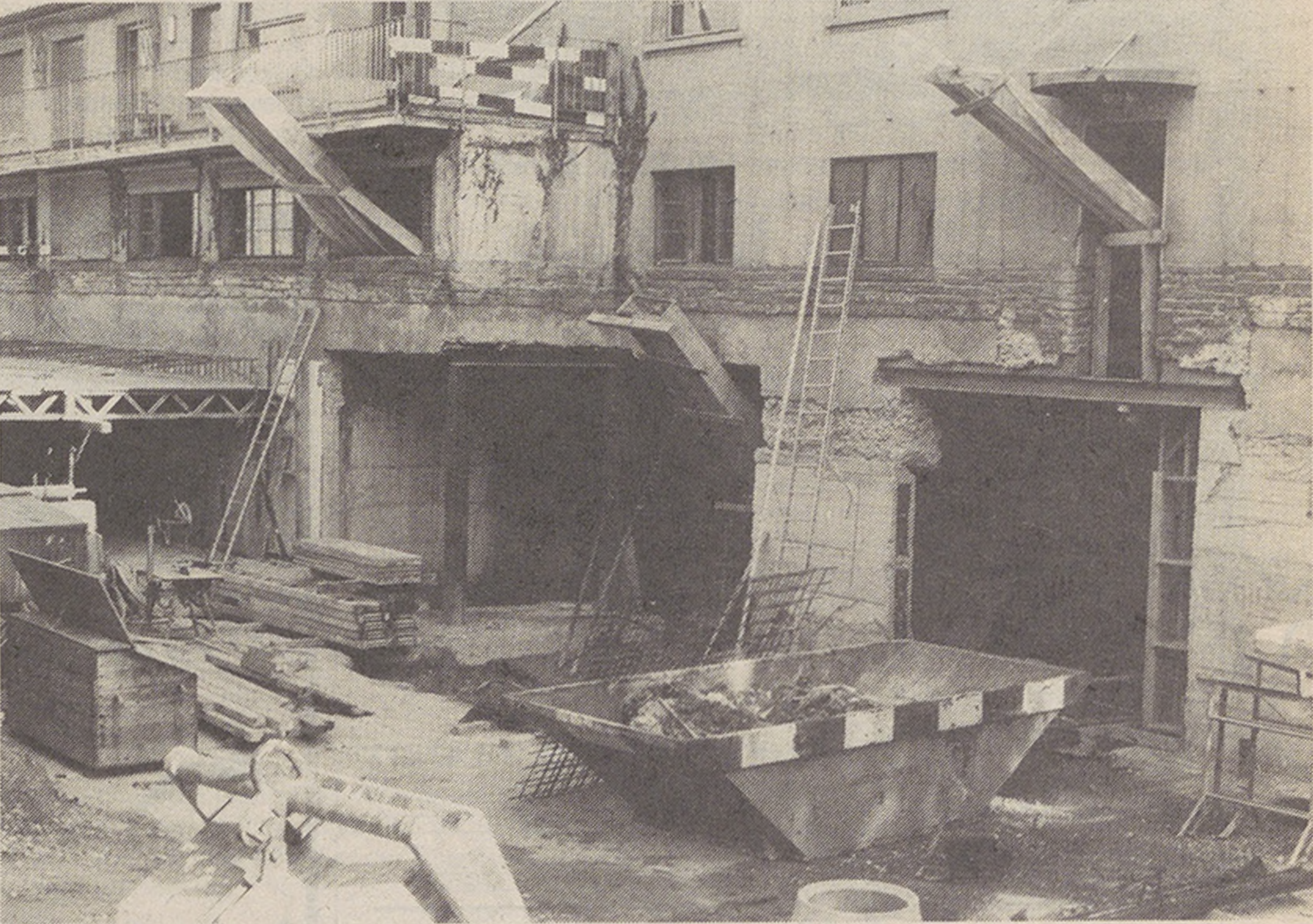
Die Unterfangung ist fertig (August 1986). Das Treppenhaus zum Garage-Geschoss, unter dem bisherigen Keller, ist ausgehoben und durch zwei dunkle Löcher erkennbar; hier werden später die Türen zur Garage (rechts) und zum Luftschuttkeller (links) gebaut.
