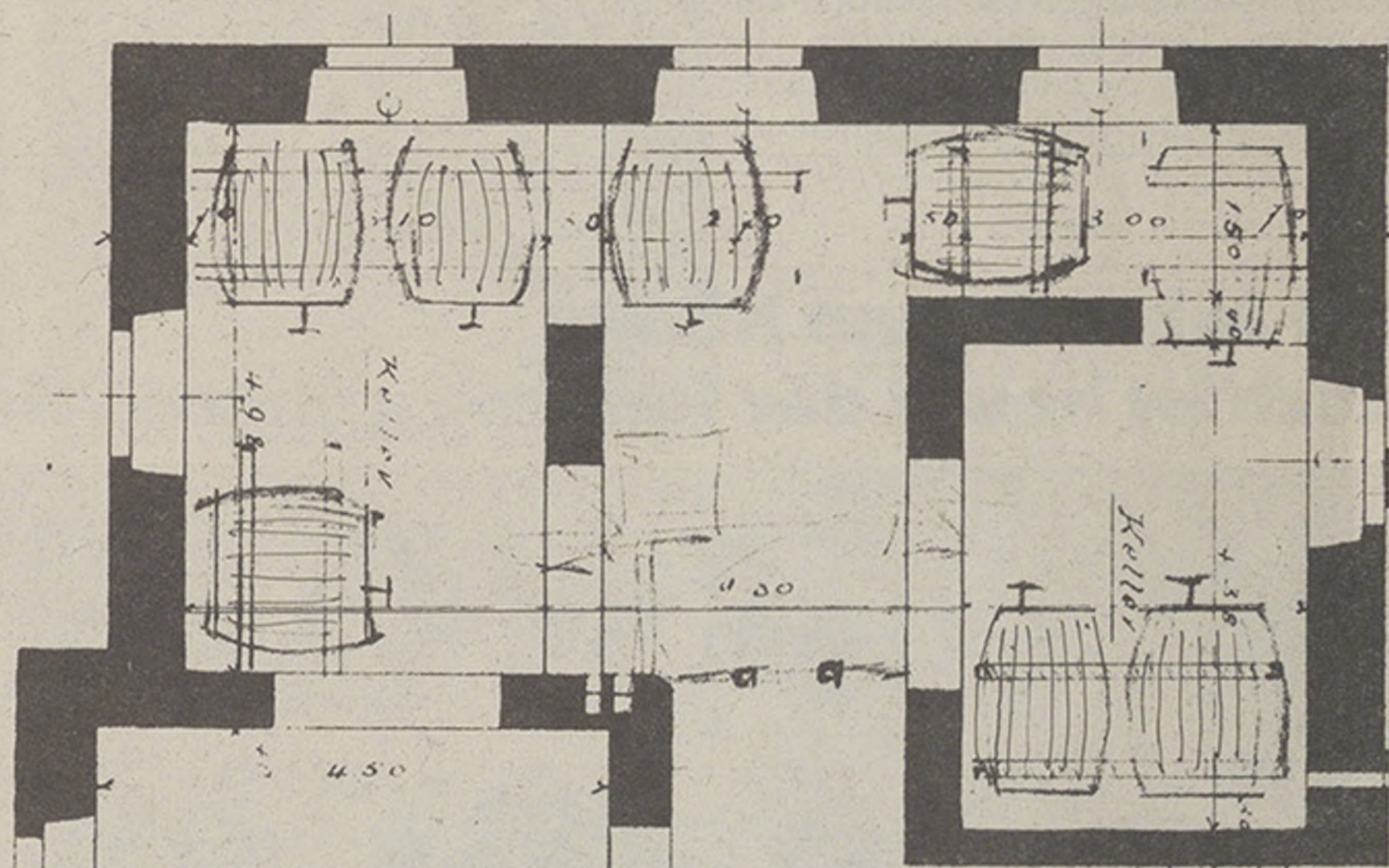
Abb. 5: Der ursprüngliche Keller mit eingezeichneten Fässern.
