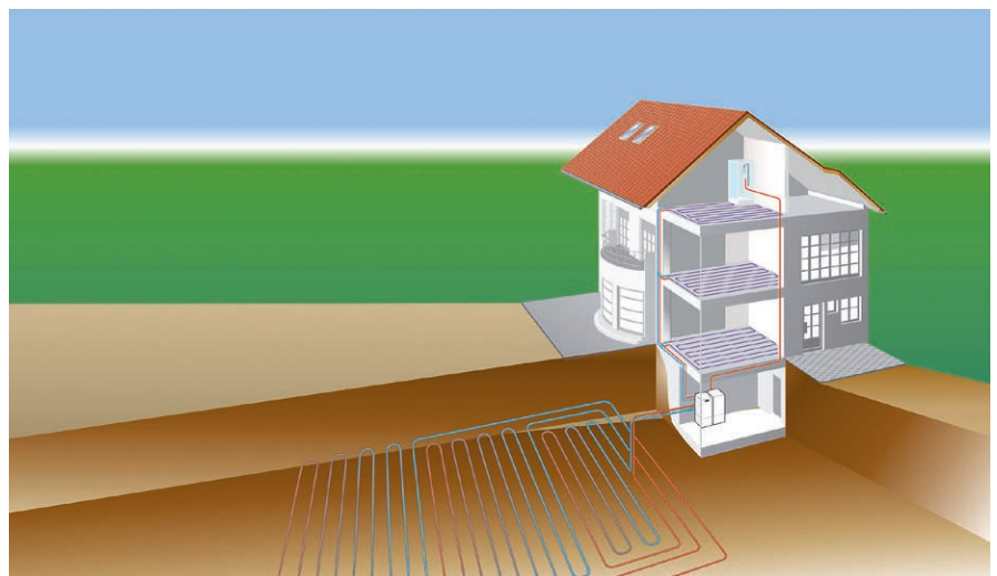
Schematisches Beispiel für eine Sole-/Wasser-Wärmepumpe mit Erdsonden (oben) und Erdkollektoren (unten)
