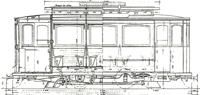
Fig.5. Elévation
