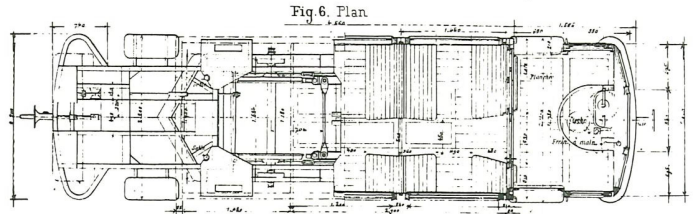
Fig.5 et 6. Automotrice à Voyageurs à deux essieux
