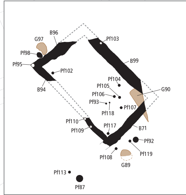
Baubefund 6 (Phasen 1 und 2), M. 1:75
