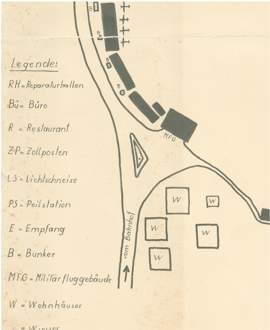
Ausschnitt des für den Vortrag im Format A2 gezeichneten Lageplanes.
