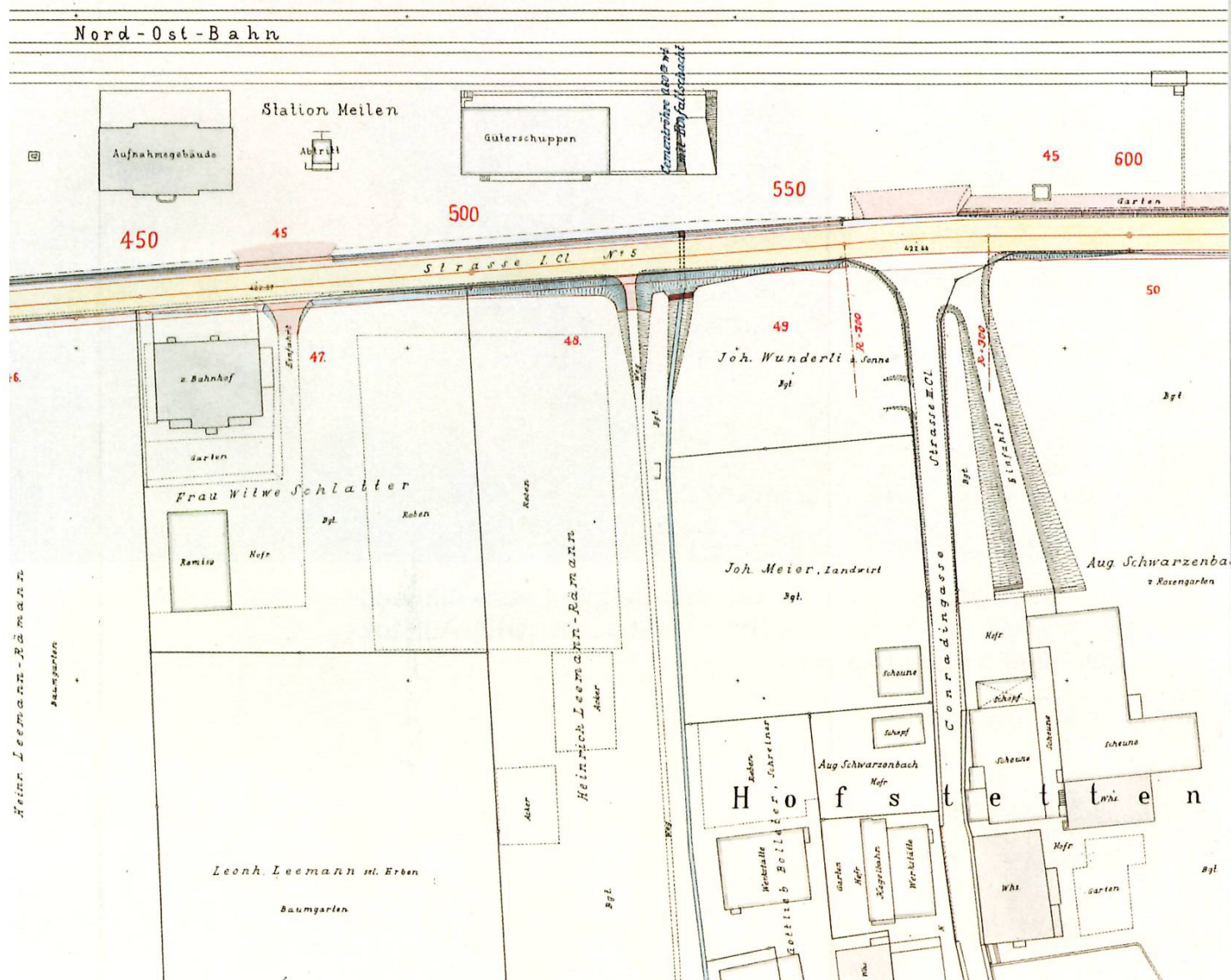
Projektplan, Originalmassstab 1:500, betreffend Korrektion der Dorfstrasse (damals Alte Landstrasse), Aufnahme um 1895.
