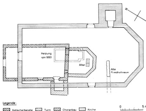
Herrliberg – Reformierte Kirche. Baugeschichtliche Untersuchungen 1962. Bauetappenplan 1 : 250.
