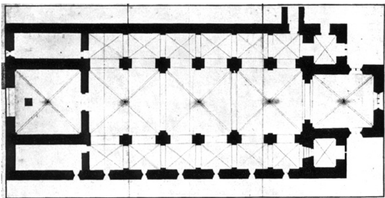
Rüti – Ehemalige Klosterkirche. Der Grundriss der dreischiffigen Basilika vor dem teilweisen Abtrag im Jahre 1770. Originalplan im Staatsarchiv Zürich.
