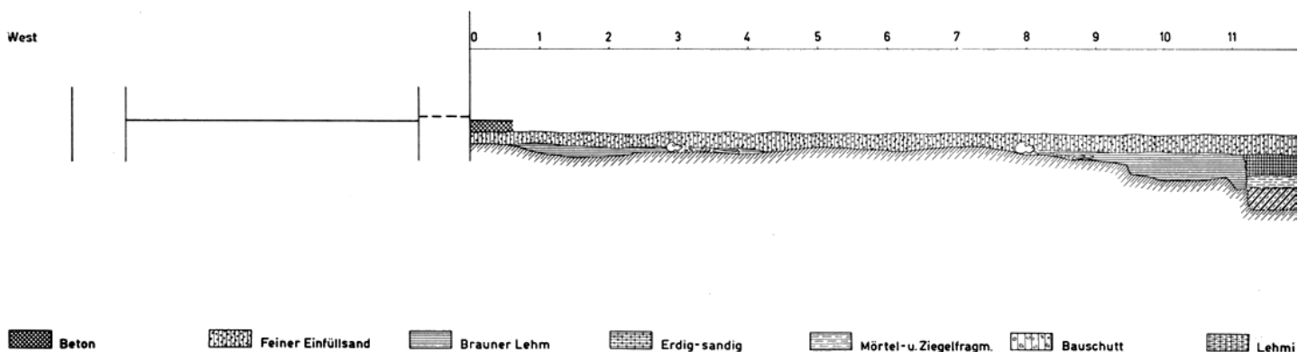
Männedorf – Reformierte Kirche. Das grosse Längsprofil A–B gemäss Planbeilage 6, 3.
