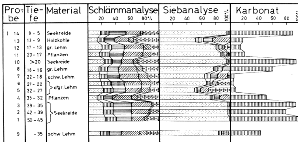
Enge – Breitingenstrasse. Neolithische Strandsiedlungsreste. Diagramm der Sedimentanalysen aus Profil A–B.
