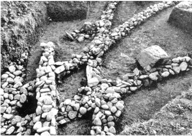
Altstetten – Loogarten. Römischer Gutshof. Reste von Drainageanlagen (?) in den Schnitten S 10 bis S 52.
