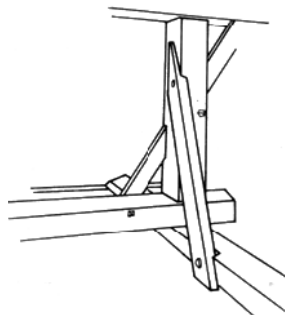
Hottingen – Zeltweg 69. Schnitt durch den alten, stehenden Dachstuhl im Nordwestteil des Hauses und Detailansicht der Stud A.
