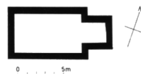
Oberglatt – Reformierte Kirche. Grundriss der ersten Kapelle, vor 1370.
