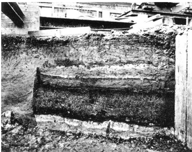
Riesbach – Utoquai. Neolithische Strandsiedlungsreste. Osthälfte des Profils A–B der Fundstelle 3 an der Hallenstrasse.
