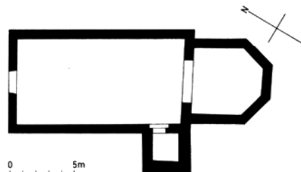
Herrliberg – Reformierte Kirche. Grundriss der um und nach 1500 um- und ausgebauten gotischen Kapelle.
