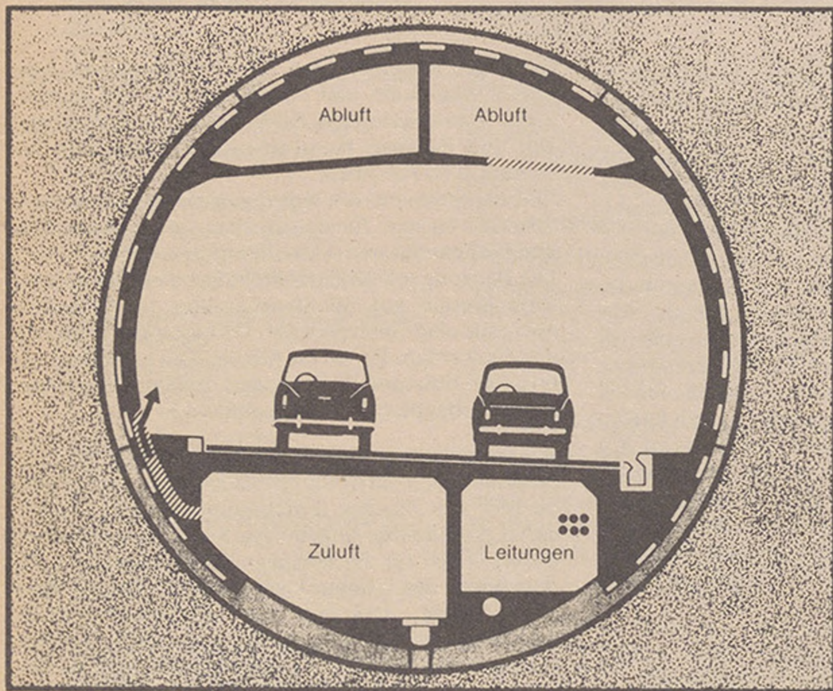
Lüftungsschema einer Tunnelröhre
