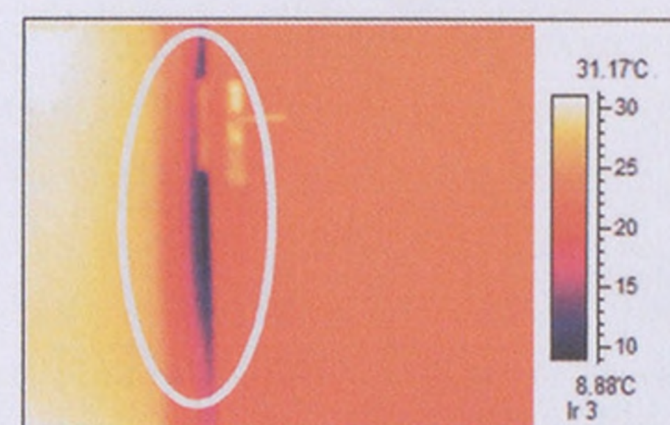
Innen: Kältebrücke bei der Haustüre Temperaturumfang Innenraum: 22°C
