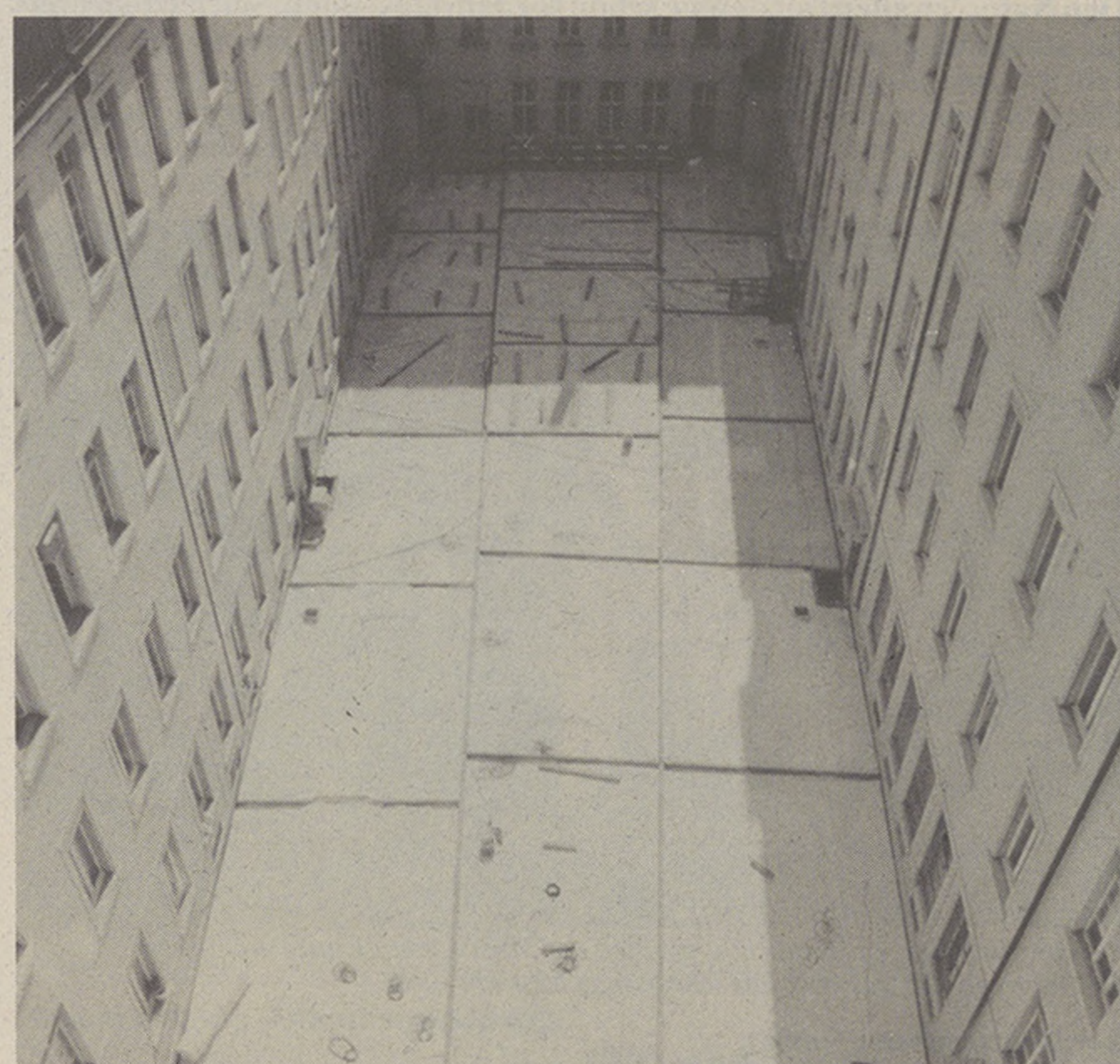
Parzellenförmig werden eine Papierschnitzelmatte und ein Metallnetz ausgelegt. Letzteres bewirkt den elektrischen Stromfluss. Die jeweiligen Anschlüsse werden an die Armierungsseisen angeschlossen.
