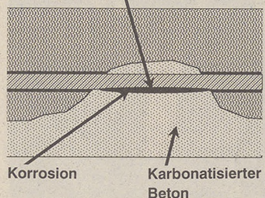
Grafik 1: Der Schaden Durch die Karbonatisierung des Betons bewirkt die Korrosion einen Abbau des Schutzmantels um die Armierung.
