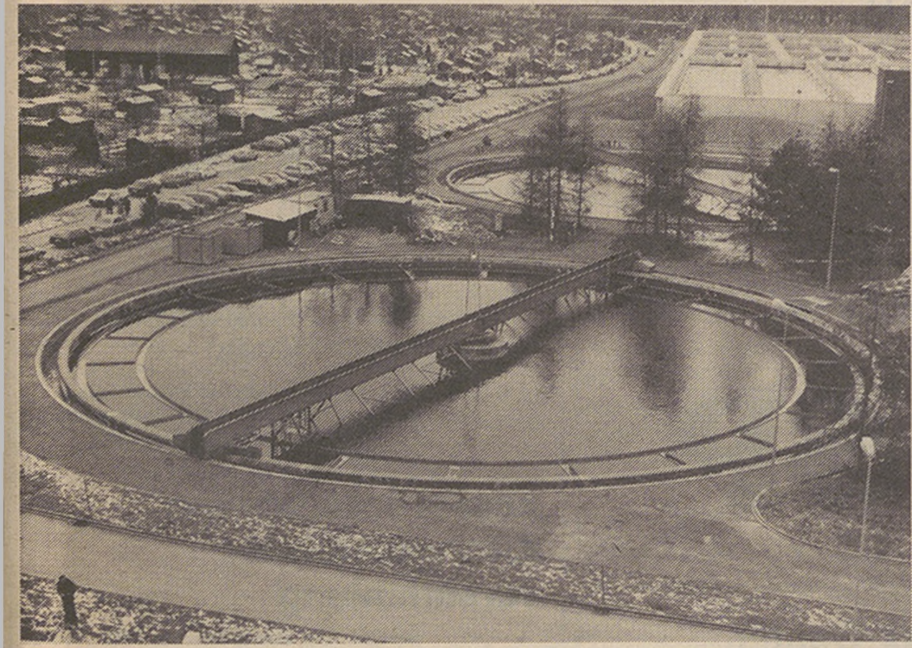
Mehrere Nachklärbecken: biologische Hauptstufe mit Hebewerk
