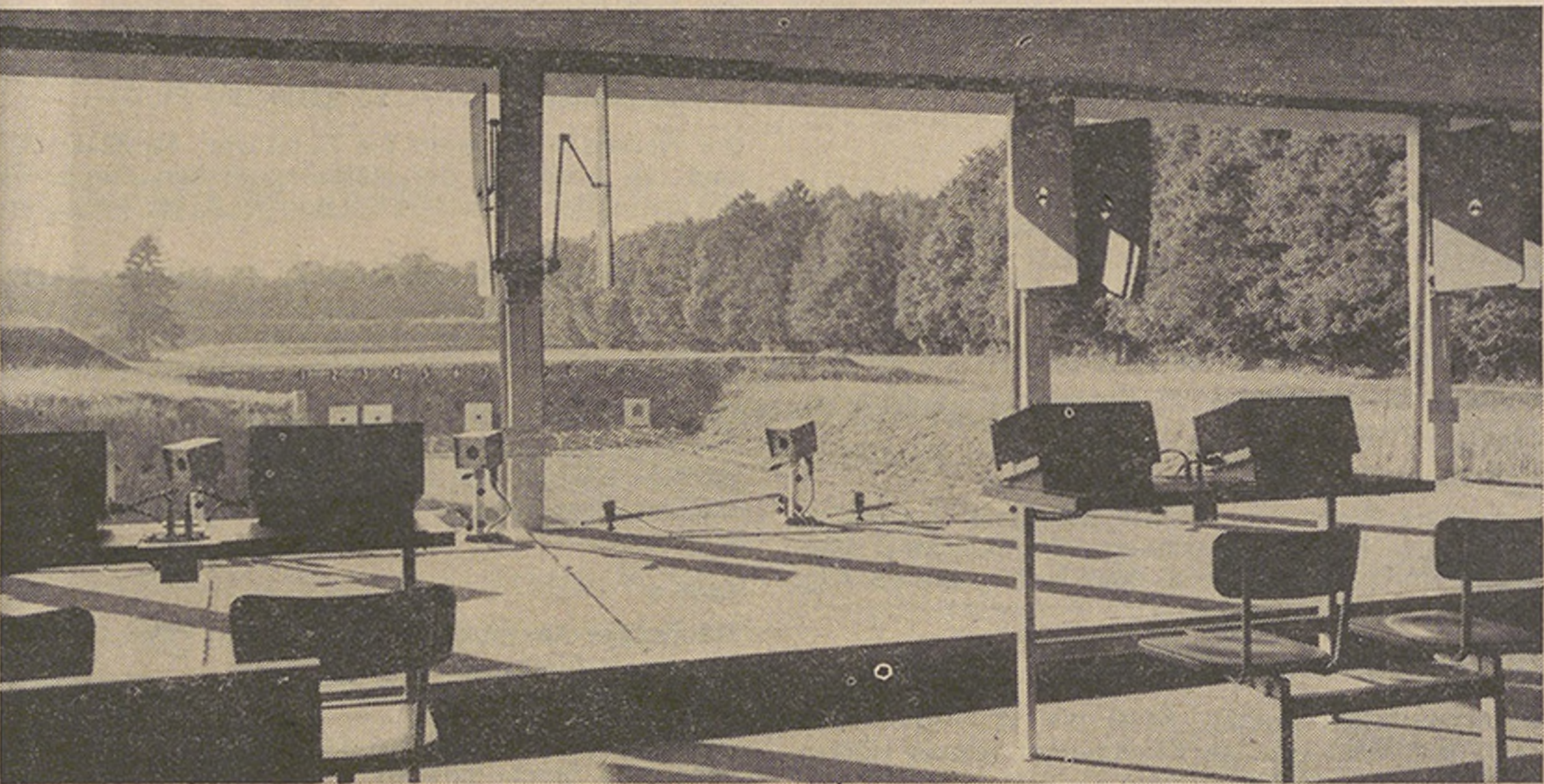
Schiessstand 300 m. Auf den Warnerpulten die Schreibautomaten der Polytronic-Trefferanzeige Unten, im Vordergrund die 50-m-Anlage mit Zugscheiben. Foto H. R. Bläsi
