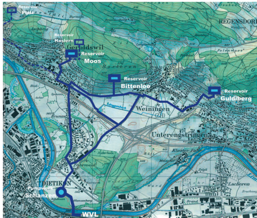
Übersicht Wassernetz-Hauptleitungen
