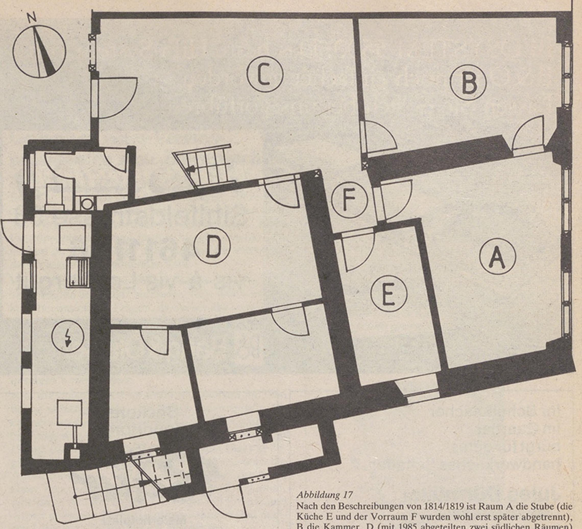
Erdgeschoss 1985 1:100
