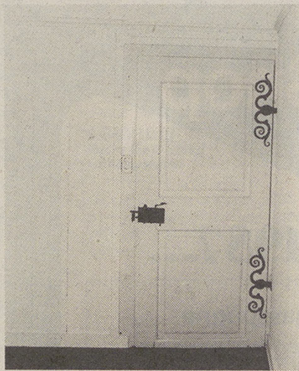
Abbildung 15 Türe im Raum H im 1. Obergeschoss, gegen Raum I; Bänder etwa Mitte 18. Jahrhundert, Schloss Ende 18. oder anf. 19. Jahrhundert. (Photo Baugeschichtl. Archiv der Stadt Zürich)
