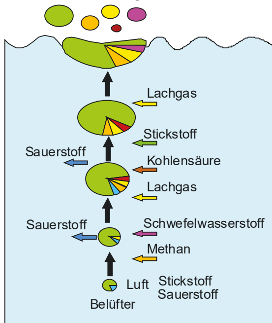
Schema der aufsteigenden Gasblasen
