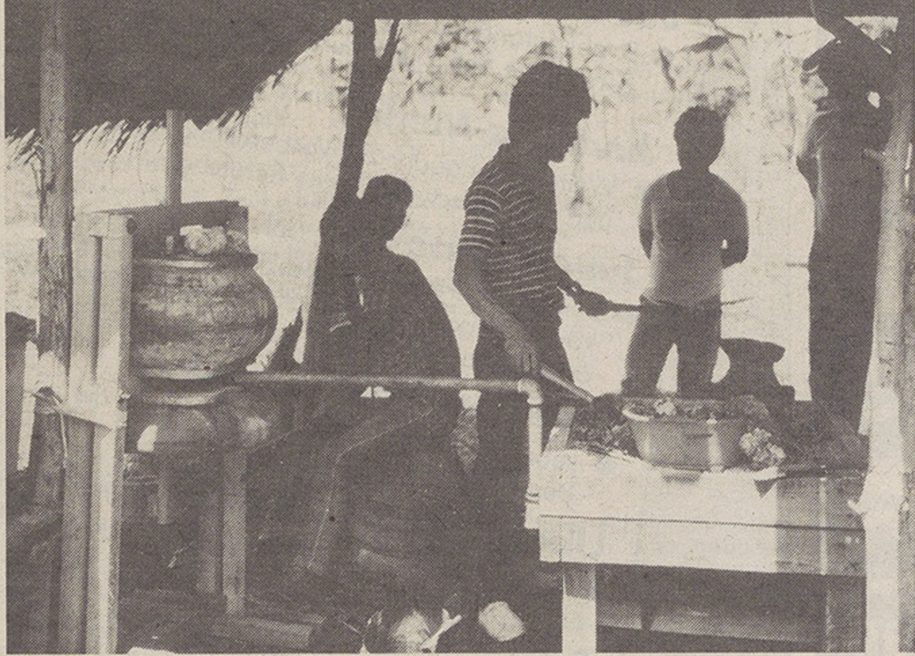
Versuchsstation für Angepasste Technik, Lapu Lapu-City. Hier wird den Kursteilnehmern gezeigt, wie mit lokalen Mitteln eine einfache Schmiedewerkstätte eingerichtet werden kann. Der Blasbalg besteht aus einem alten Autodach.
