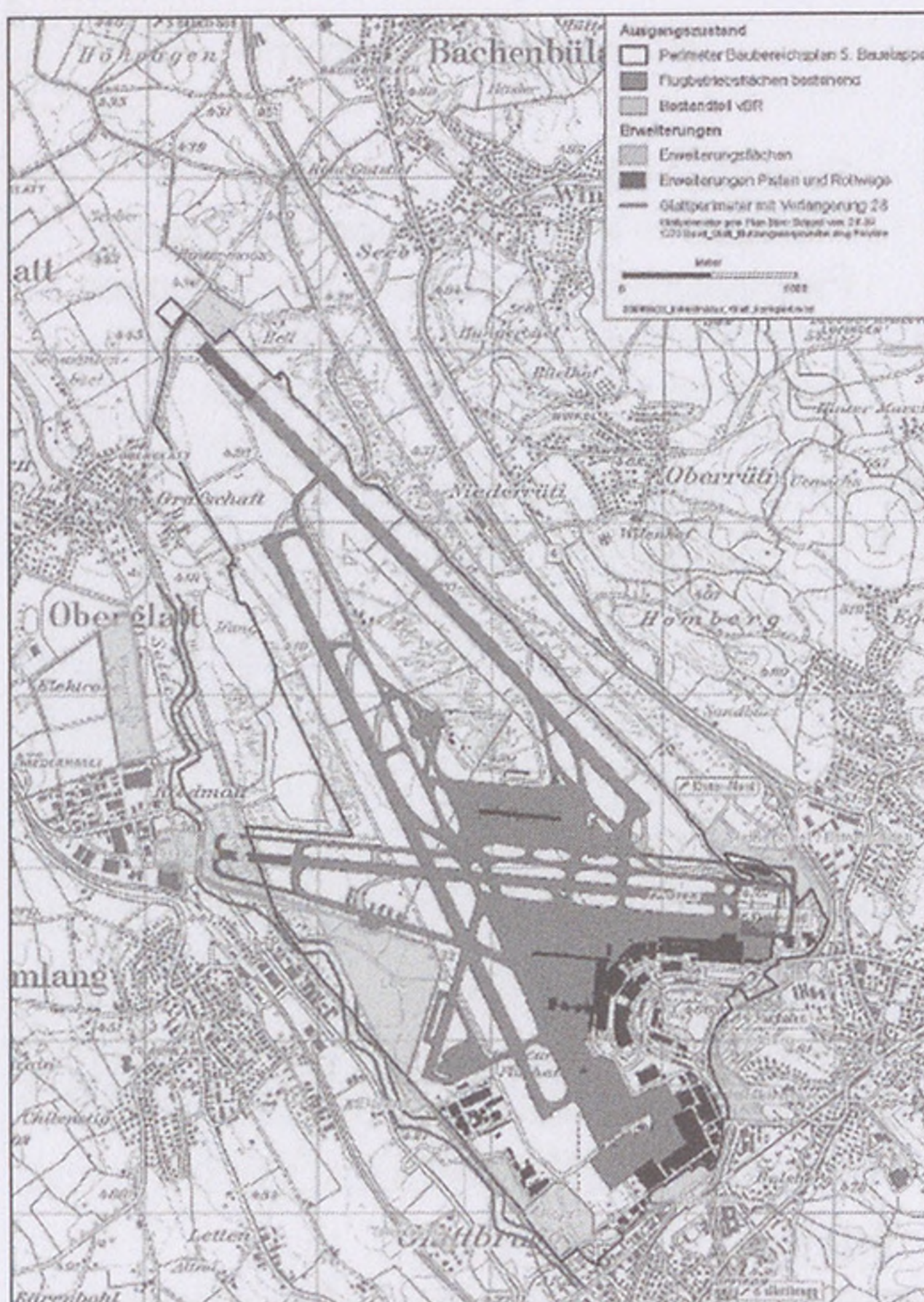
Objektblatt 3b SIL-Entwurf vom 16.8.10: Infrastrukturanlagen mit Pistenverlängerungen 28 und 34.
