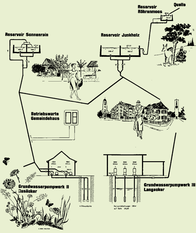
Das Schema der Wasserversorgung Dietikon von 1957 ist ein grafischer Leckerbissen. Es zeigt Dietikon noch als Dorf, umgeben von viel Natur. Die Anlagen der Wasserversorgung sind aber bereits für ein Gross-Dietikon mit gegen 25 000 Einwohnern konzipiert.
