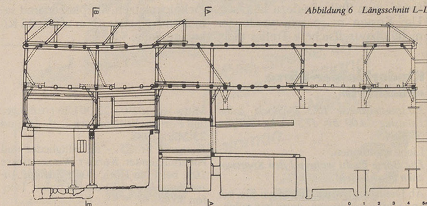
Abbildung 6 Längsschnitt L-L
