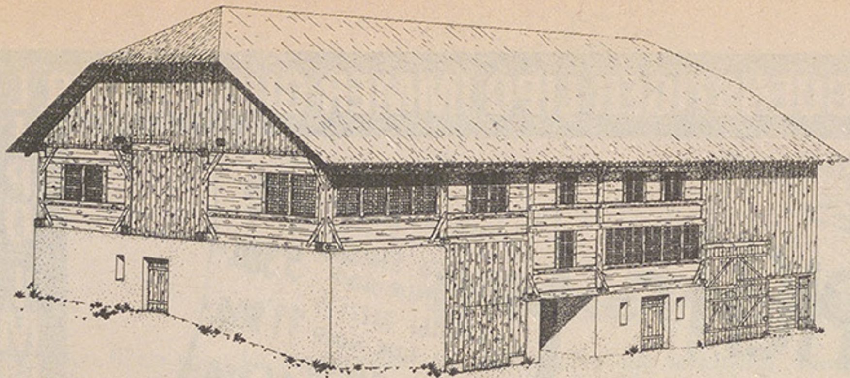
Abbildung 9 Rekonstruktionsversuch des Hauses in seinem vermutlichen Zustand um 1550; Links (erste zwei Fenstergruppen der Längswand) Anbau von 1544 (= hinteres Haus), in der Mitte der Wohnteil von 1538 (zwei hölzerne Wohngeschosse über gemauertem Sockelgeschoss), rechts der Scheunenteil von 1538 (ganz aus Holz).
