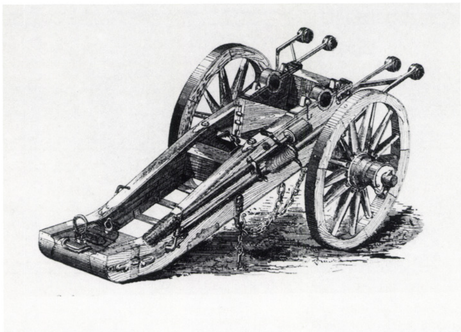
Lafette einer Kanone (aus: Dolleczeck. Geschichte der österreichischen Artillerie)
