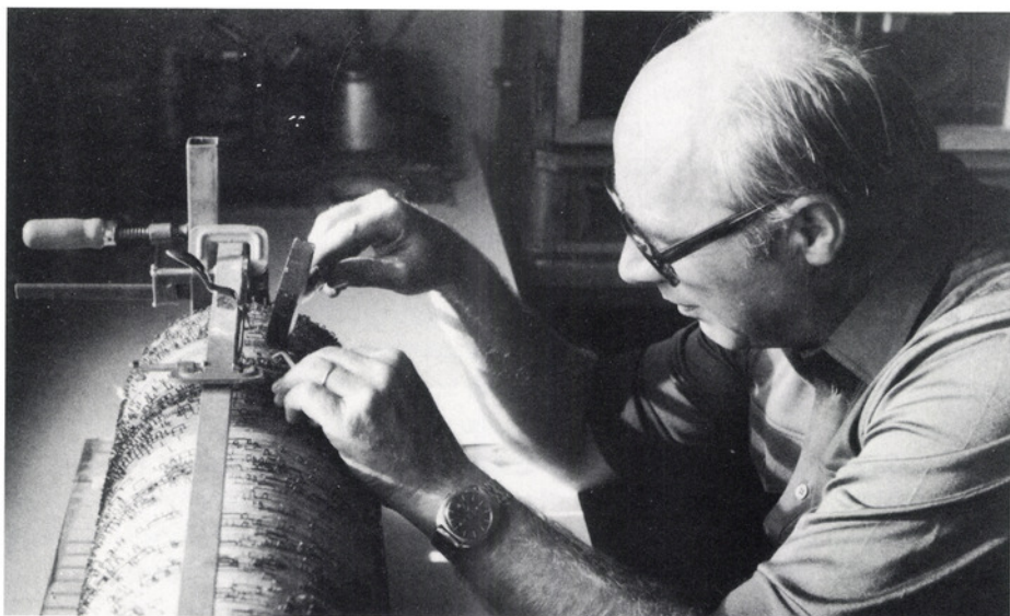
Werner Tschudin revidiert eine Stiftenwalze; eine äusserst arbeitsintensive Tätigkeit, die eine ruhige Hand braucht
