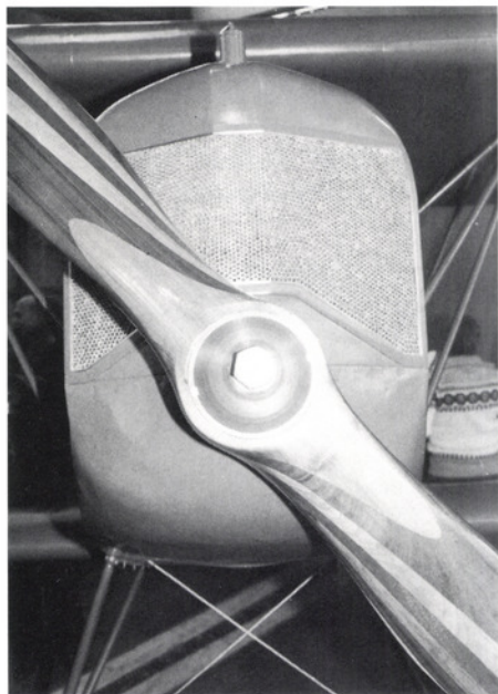
Bis ins letzte Detail genau nachgebaut sind Kühler und Propeller
