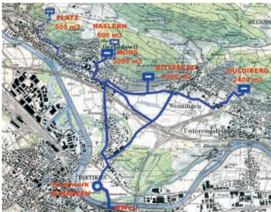
Übersichtsplan Gruppenwasserversorgung GOW – Geroldswil-Oetwil-Weiningen
