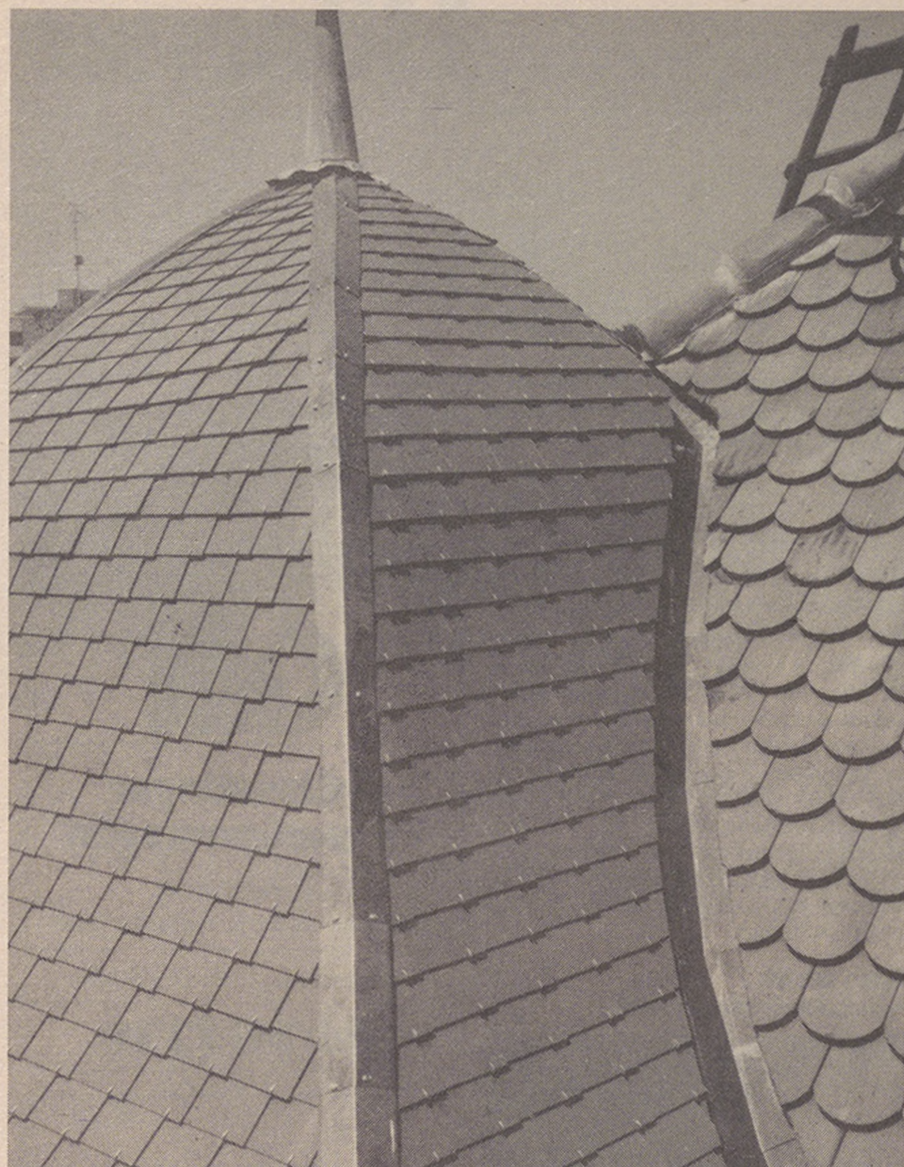
Das Bild zeigt die Dacheindeckung eines Erkers mit Faserzementplatten als geschlufte Deckung. Faserzementplatten sind das geeignete Material für geschweifte Dächer.
