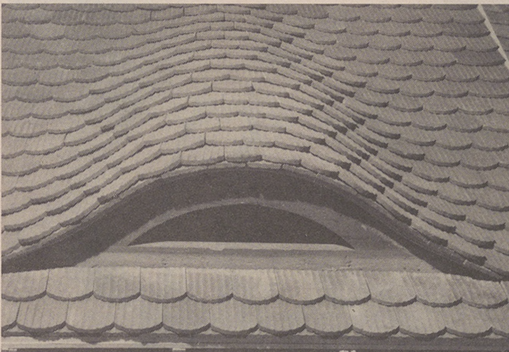
Das Bild zeigt eine Dacheindeckung mit Biberschwanzziegeln (Rundschnitt). Diese Form eines Fensters in der Dachfläche nennt man Ochsenauge oder Fledermausgaube.
