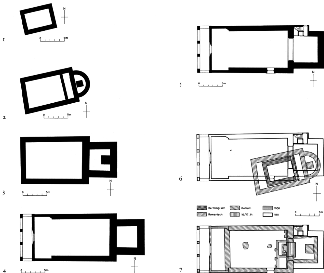
Fehraltorf. Reformierte Kirche. Bauetappenpläne: 1 Karolingisch, 2 Romanisch, 3 Gotisch, 4 Nach dem Umbau 1906, 5 Nach dem Turmbau 1911, 6 Gesamtplan mit Bauetappen 1 und 2, 7 Gesamtplan mit Bauetappen 3 und 4. Mst. 1:400.
