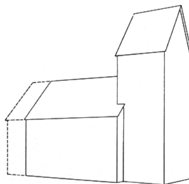
Fehraltorf. Reformierte Kirche. Rekonstruktion der Bauetappen 1–3.
