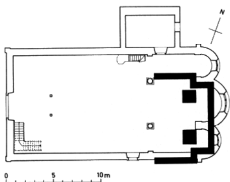
Rheinau. Bergkirche St. Nikolaus. Bautappenpläne: 1 Romanisch, 2 mit Chorschränkenmauern, 3 nach Einbau von Pfeilern. Weiss gehaltener Grundriss: Bau von 1578/79. Mst. 1:250
