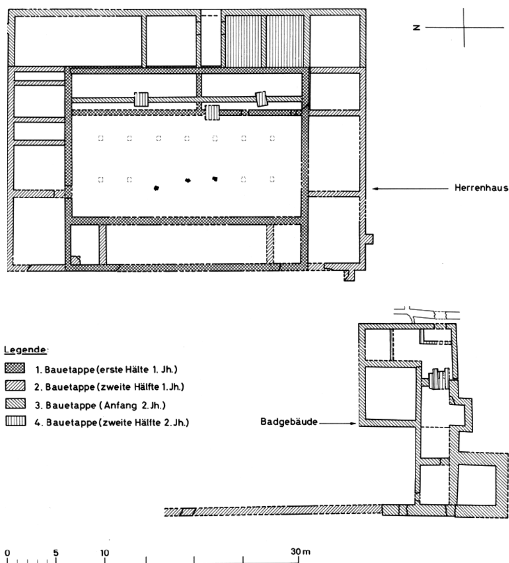
Urdorf, Heidenkeller/Unterer Keimler. Herrenhaus und Badegebäude eines römischen Gutshofes. Bauetappenplan.
