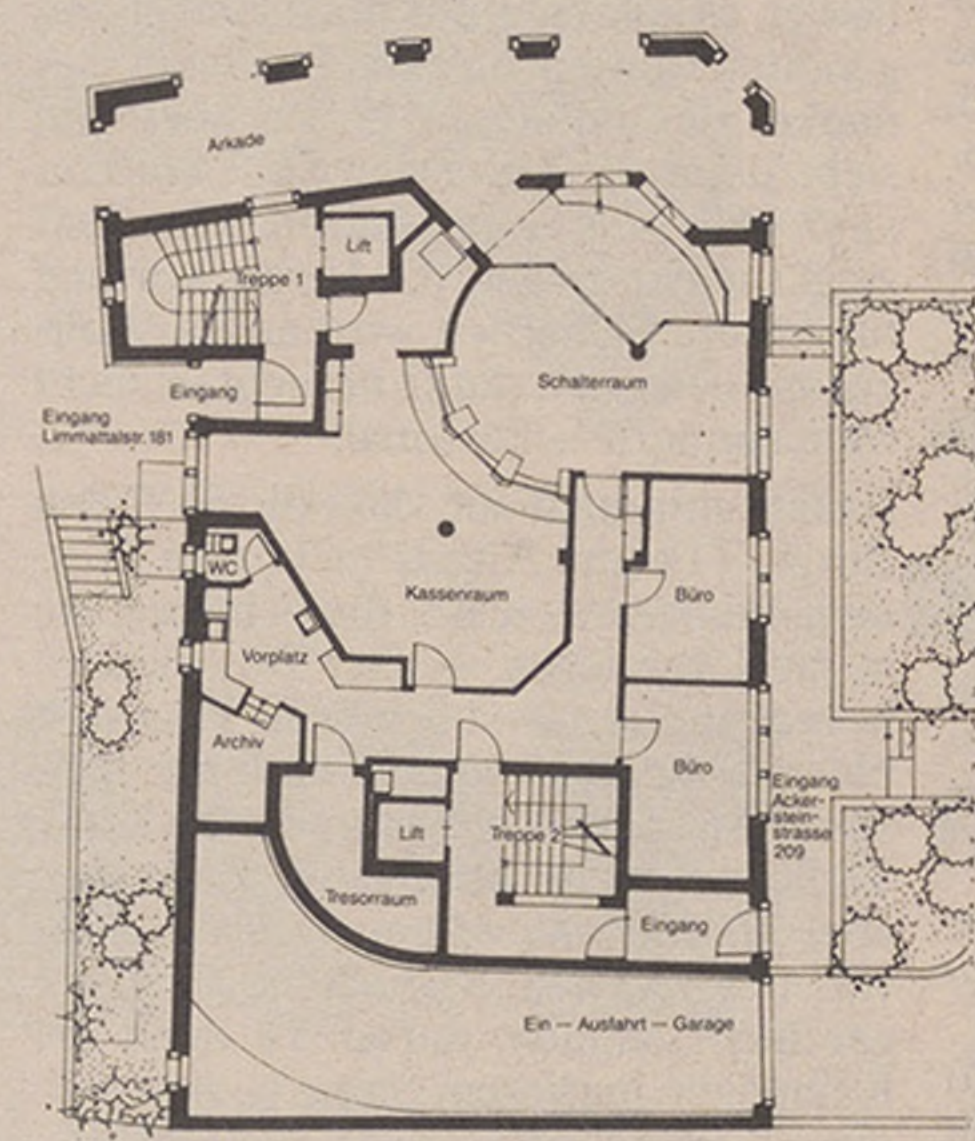
Abbildung 32 Grundriss Erdgeschoss Neu-bau vorderes Haus
