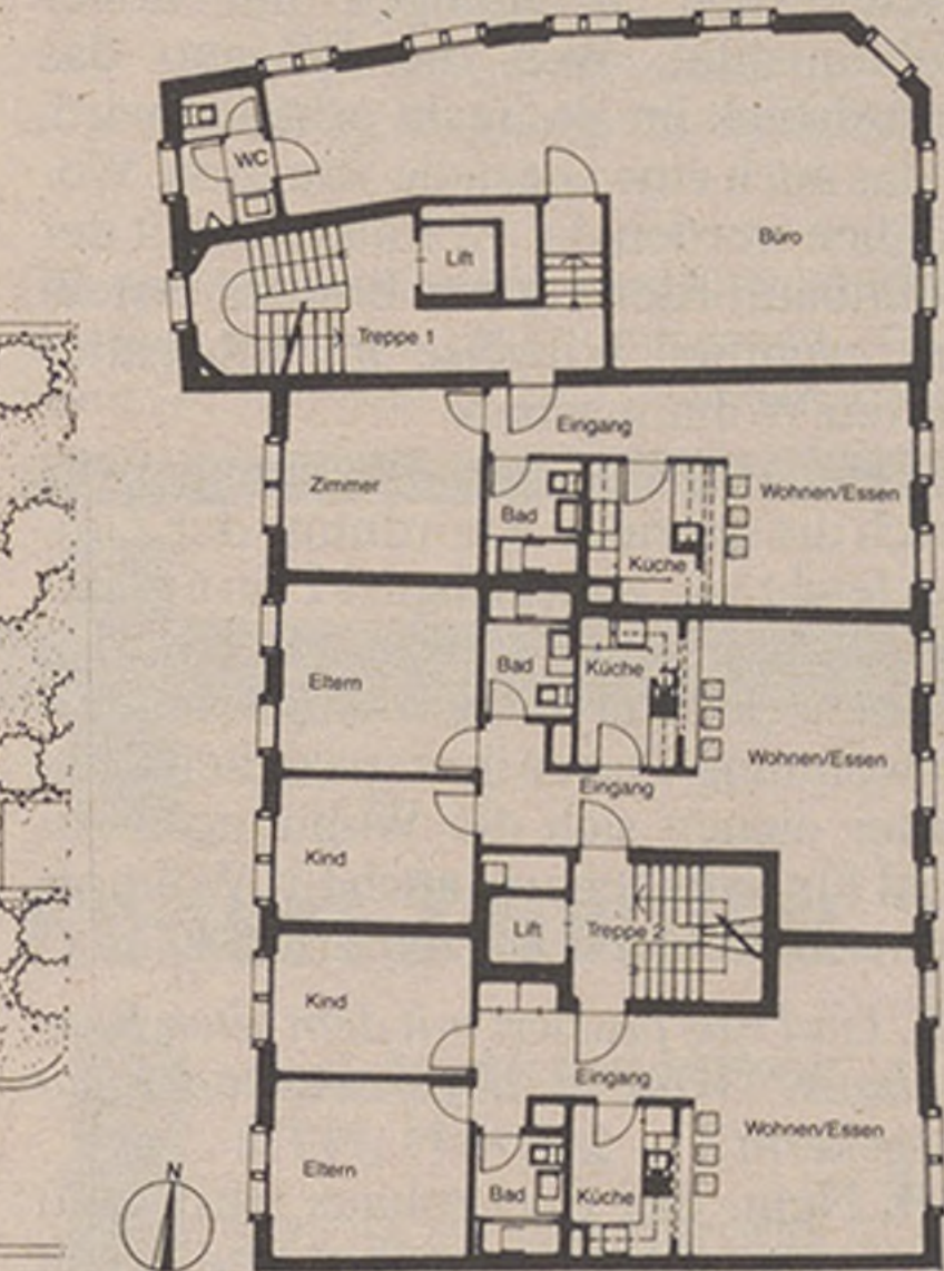
Abbildung 33 Grundriss zweites Ober-geschoss Neubau vorderes Haus
