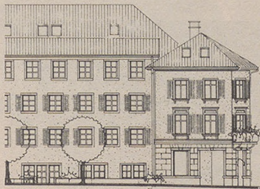
Abbildung 30 Ostfassade Neubau vorderes Haus
