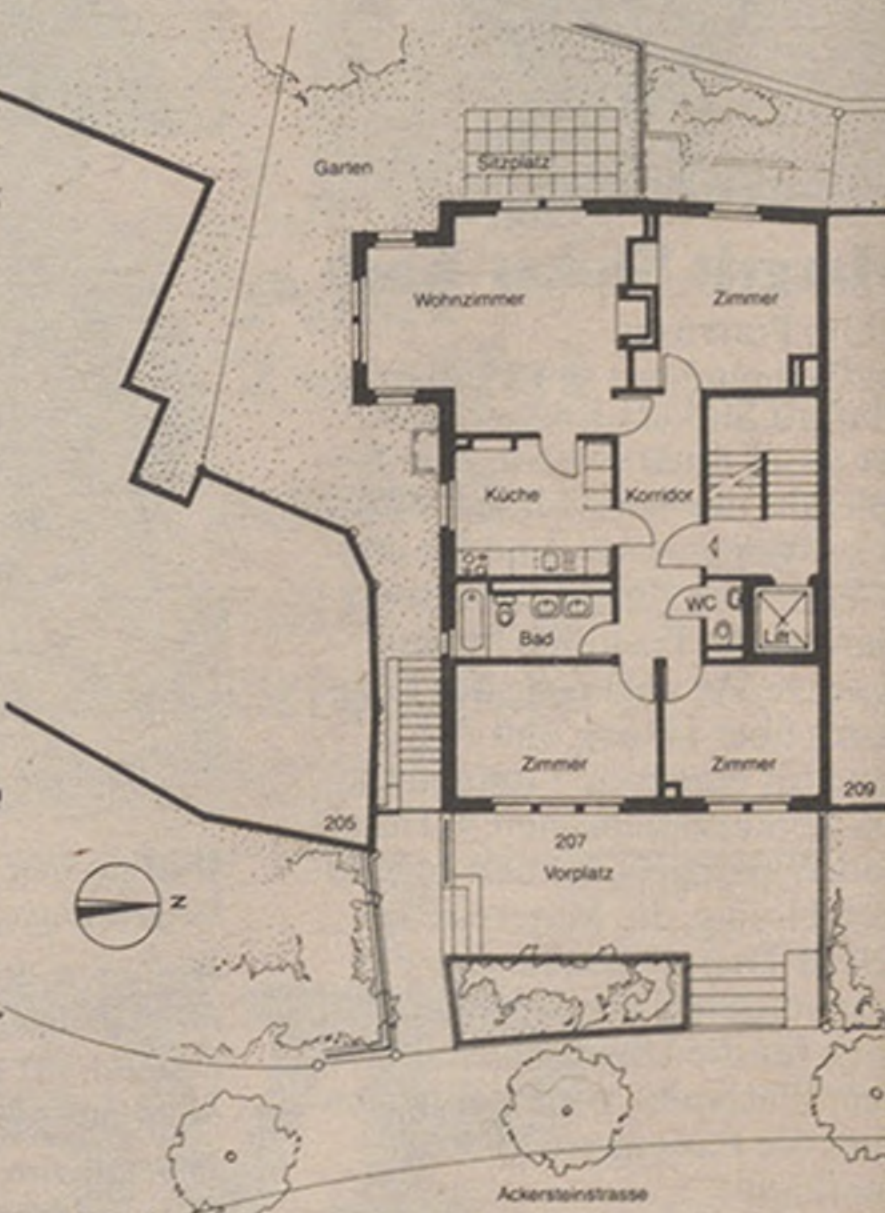
Abbildung 39 Grundriss Erdgeschoss Neu-bau hinteres Haus
