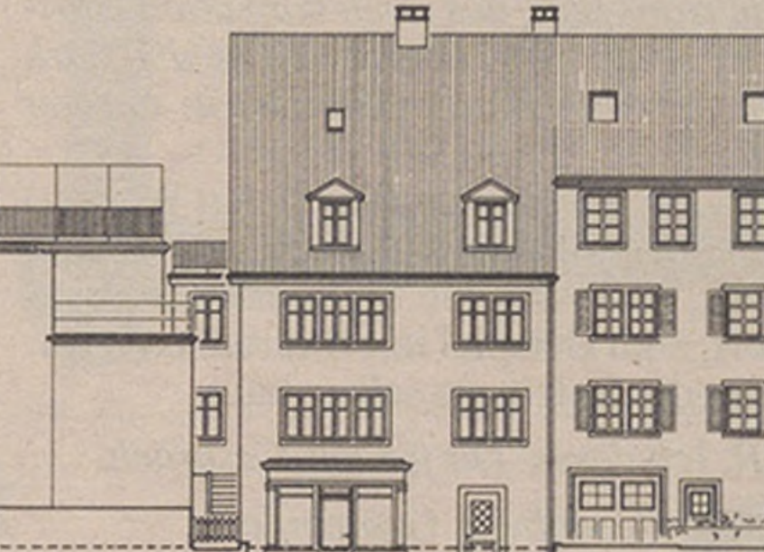
Abbildung 35 Ostfassade Neubau hinteres Haus
