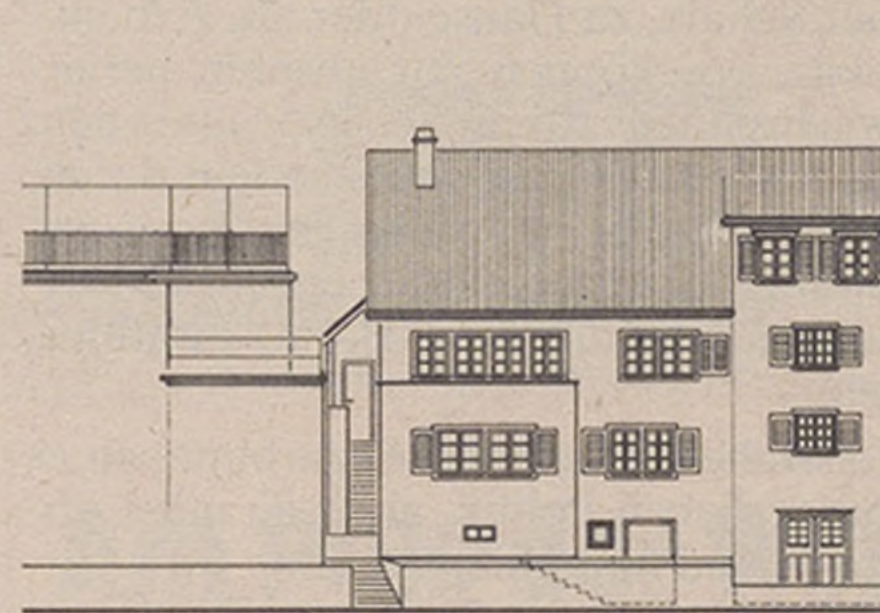
Abbildung 34 Ostfassade abgebrochenes hinteres Haus
