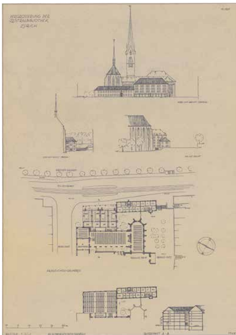
Planskizze von 1948 für einen Erweiterungsbau.
