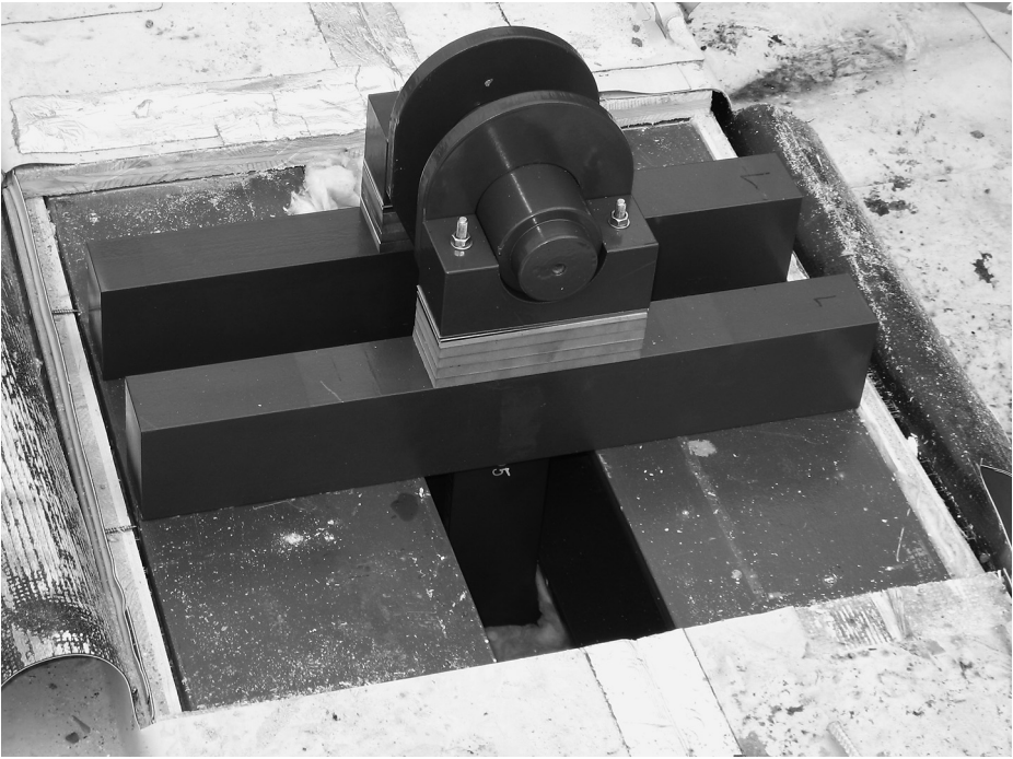
Detailansicht der CFK-Spanngliedverankerung auf dem Dach des renovierten und ertüchtigten Empa-Gebäudes.
