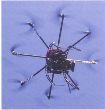
Der Oktokopter auf Grund und in der Luft, bestückt mit einer Full HD Videokamera (Bild: Doris Bruno)
