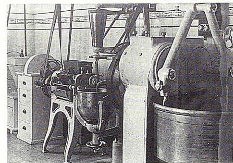
Mahl-, Walz-, Rühr- und Teigknetmaschinen an einer Transmission in der Backstube der Bäckerei Hänsele 1916.
